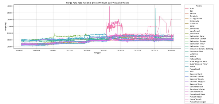
Fig. 1. Dataset
